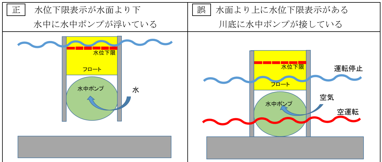
図3 (水中ポンプのフロート部の下限表示イメージ)
